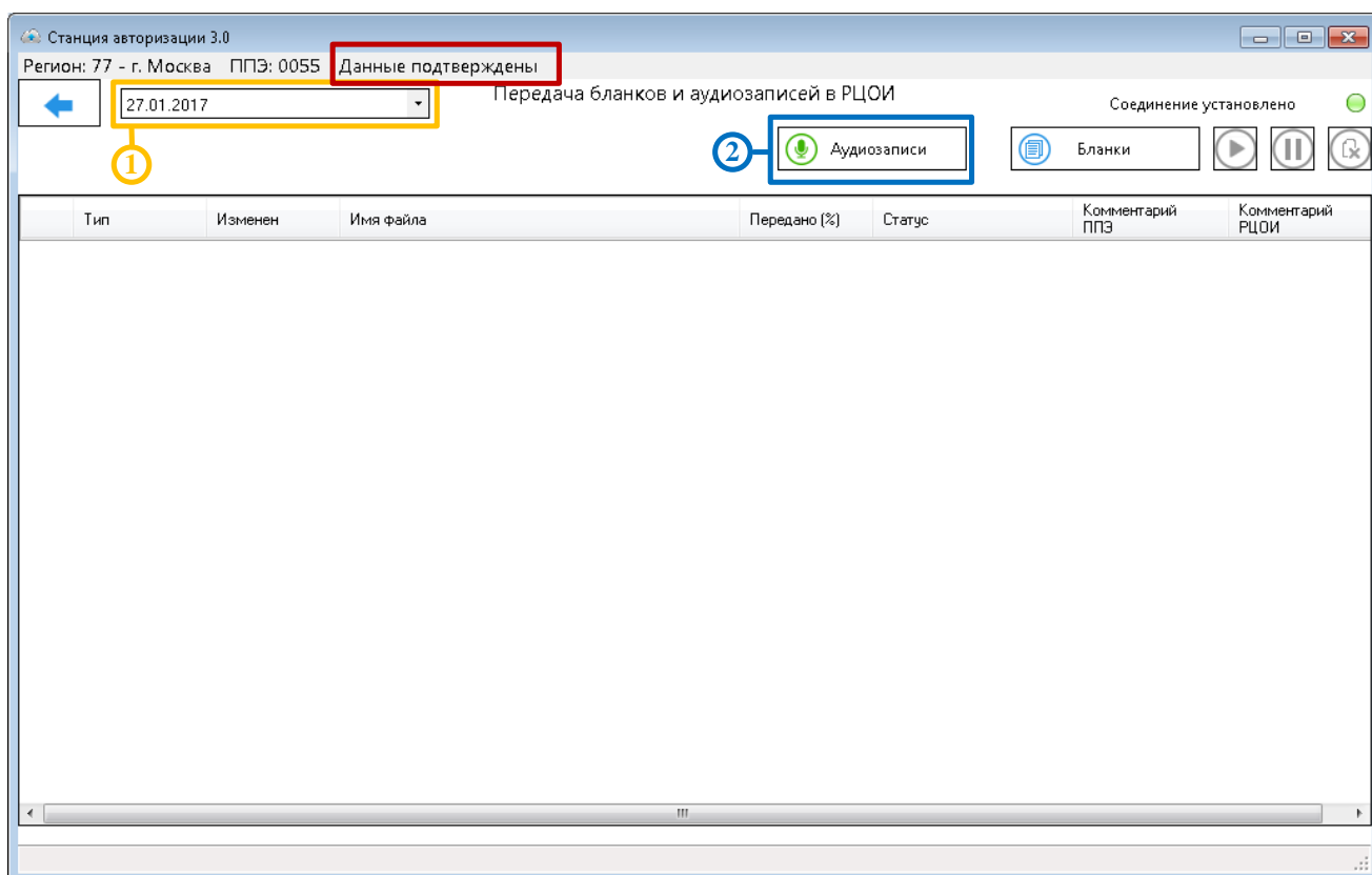
Рис. 60. Передача аудиозаписей в РЦОИ
