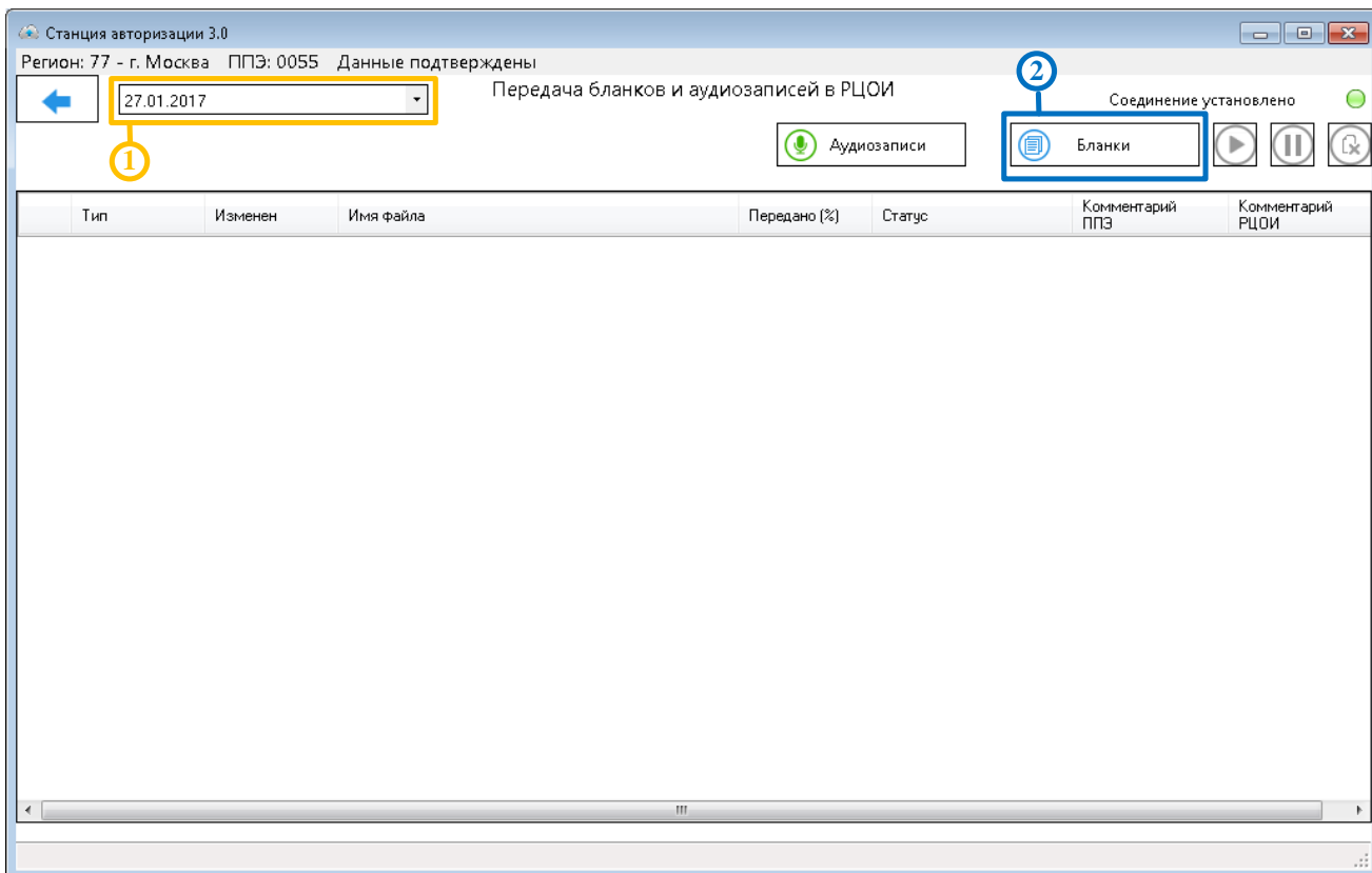
Рис. 53. Передача бланков в РЦОИ
