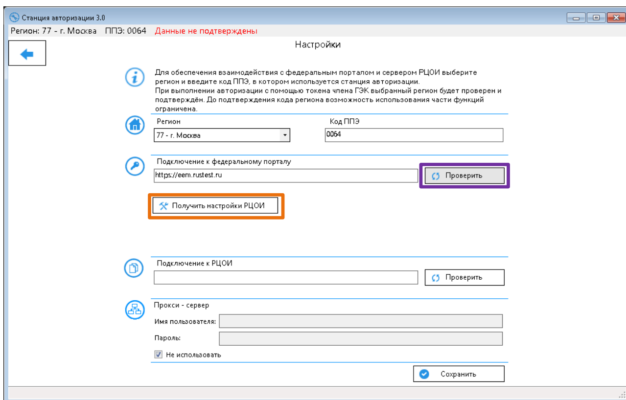
Рис. 47. Проверка подключения к федеральному portalу
