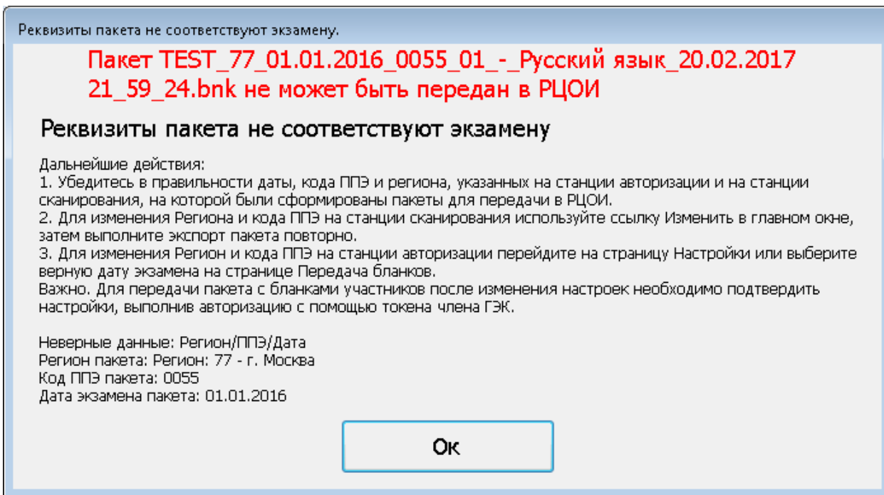
Рис. 59 Ошибка при попытке передачи пакетов с данными, не соответствующими настройкам станции авторизации.
