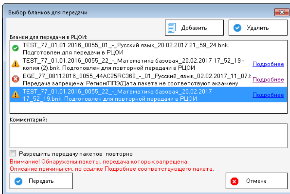
Рис. 55. Результат обработки пакетов в процессе подготовки к передаче в РЦОИ
