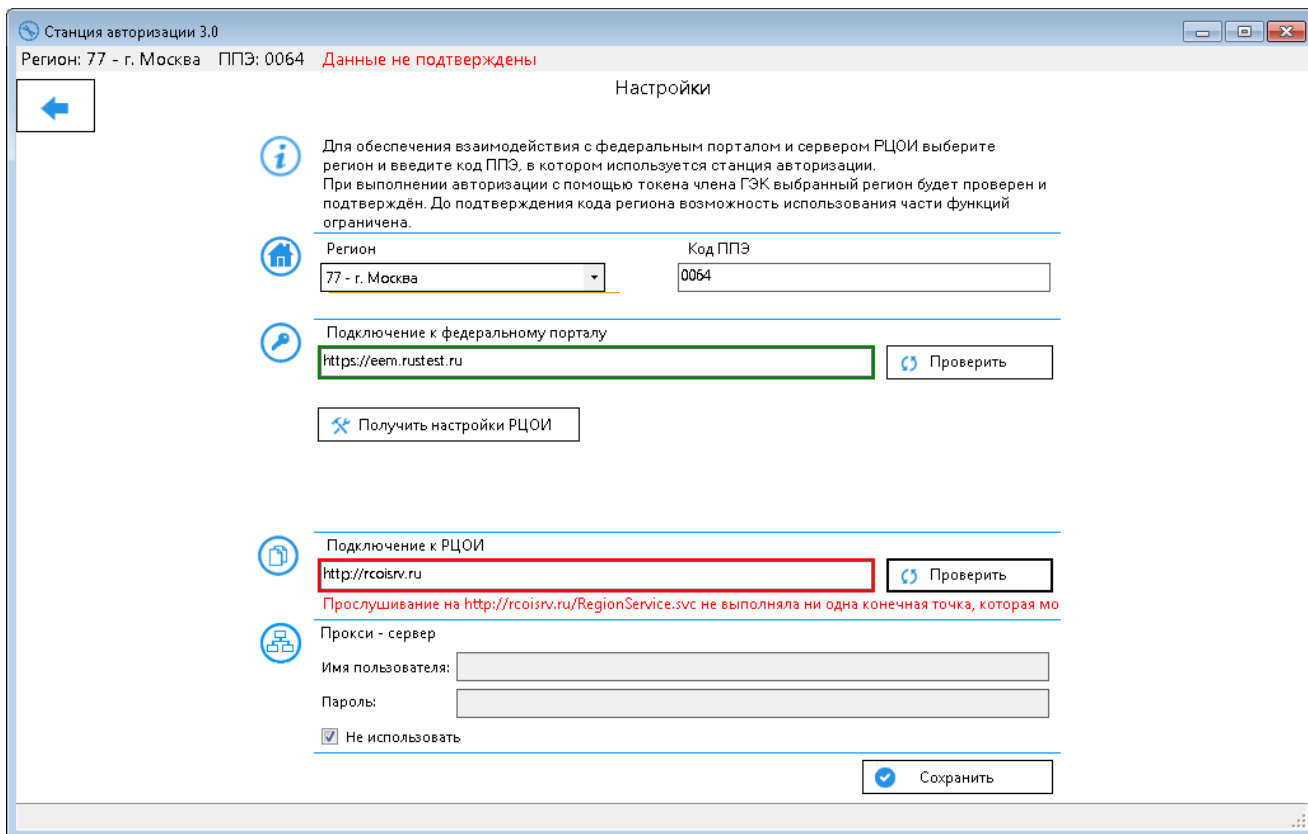
Рис. 50. Нештатная ситуация. Невозможно подключиться к серверу РЦОИ по указанному адресу.
