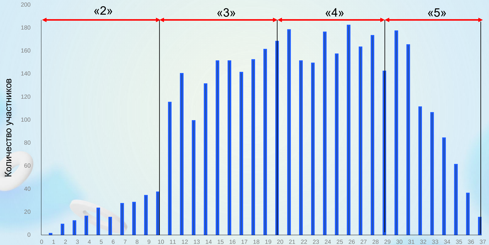
Распределение баллов
