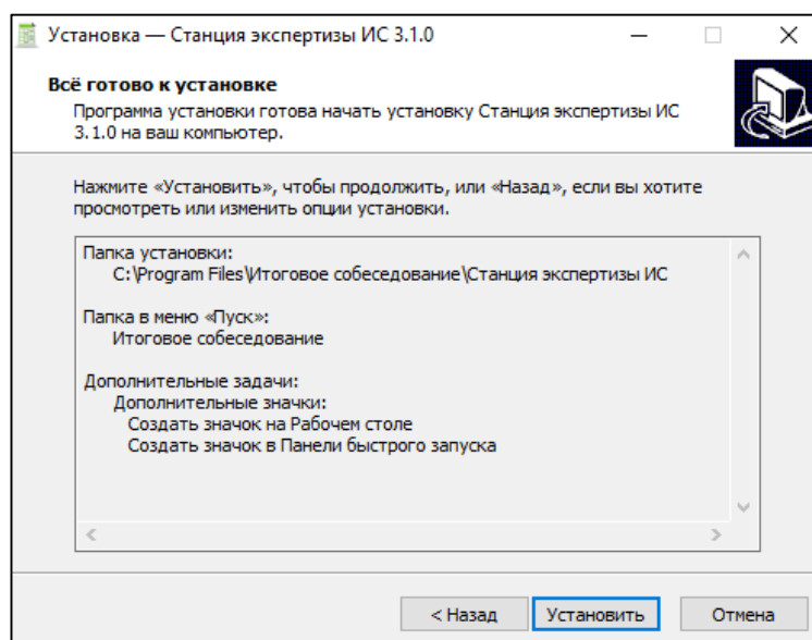
Рис. 6. Подтверждение установки
