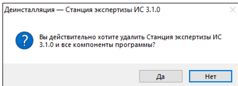
Рис. 24. Удаление программы
