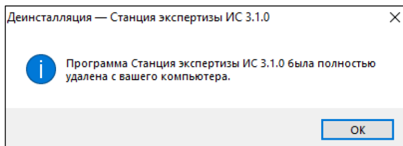
Рис. 25. Удаление программы
