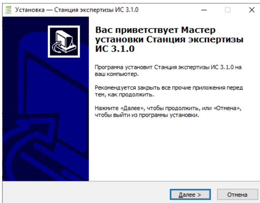
Рис. 2. Установка ПО
