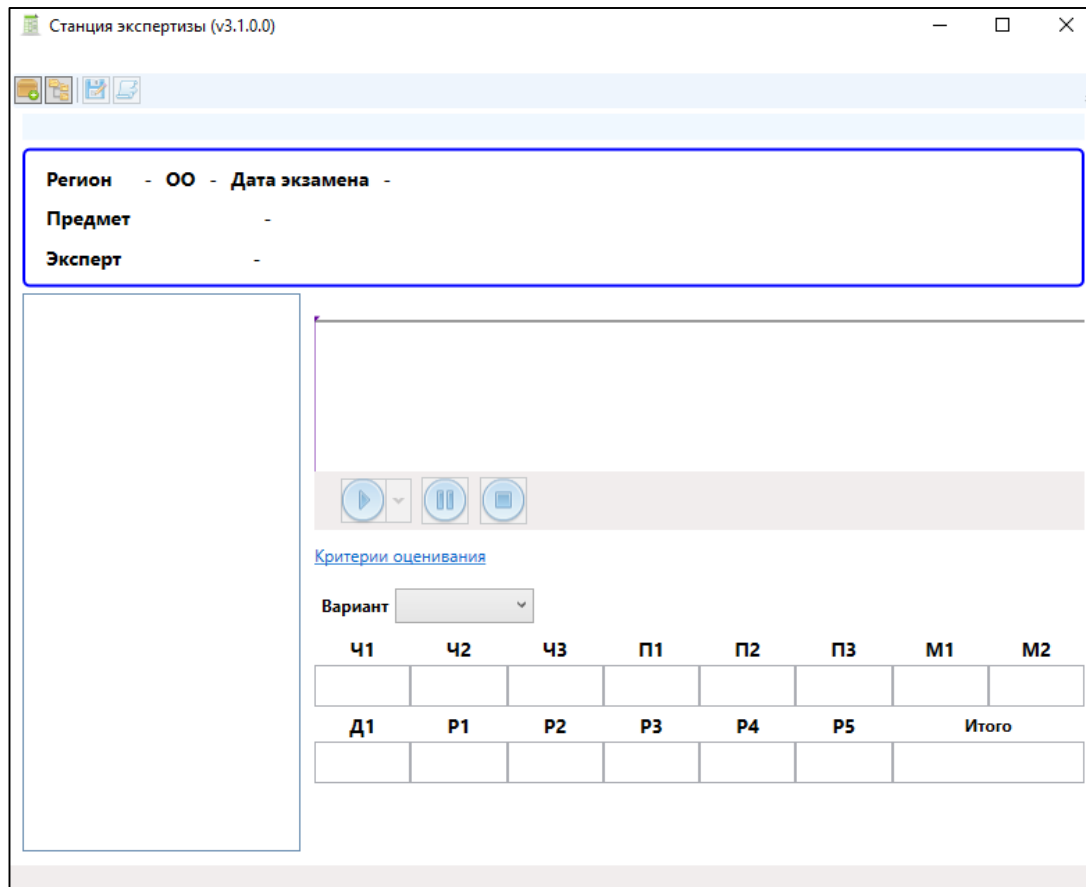
Рис. 13. Главное меню
