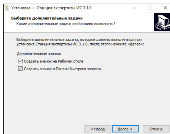
Рис. 5. Дополнительные задачи
