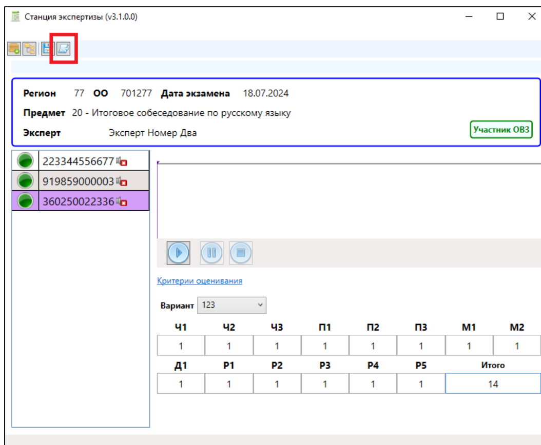
Рис. 23. Экспорт результатов
